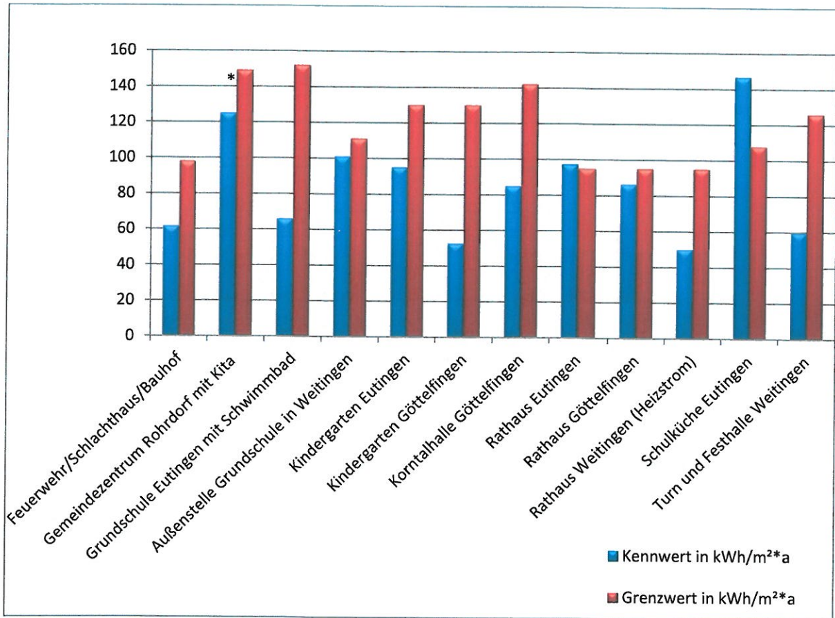
Abbildung 7: Heizenergieverbrauch (witterungsbereinigt): Kenn- und Vergleichswerte
